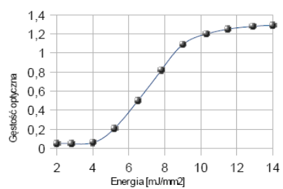
Czułość dynamiczna
